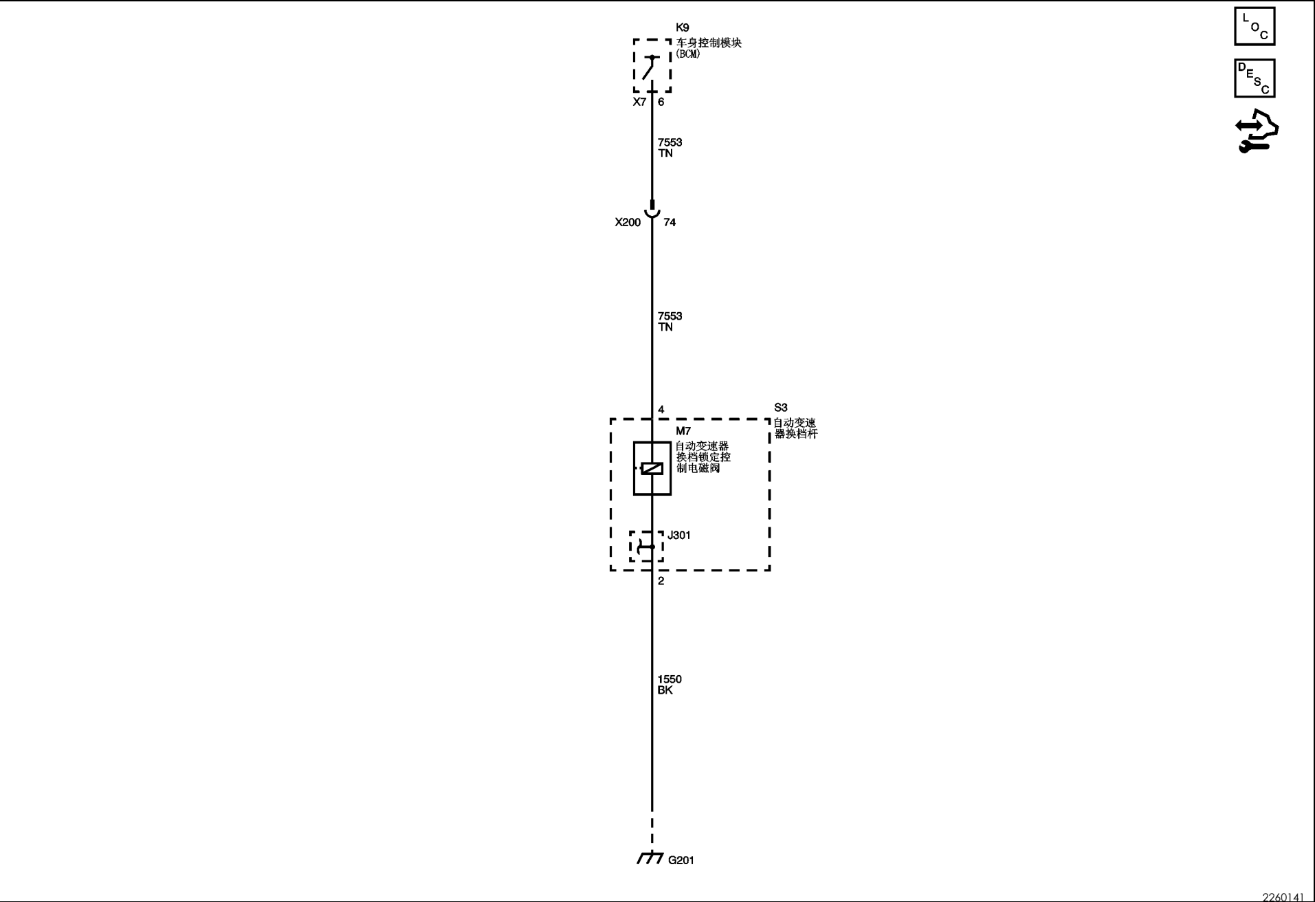
换档锁定控制示意图(换档锁定控制系统)
